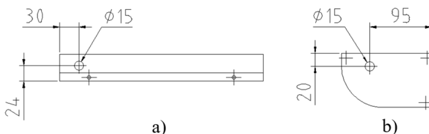
Figur 1. Plassering av hull i monteringsplate.
