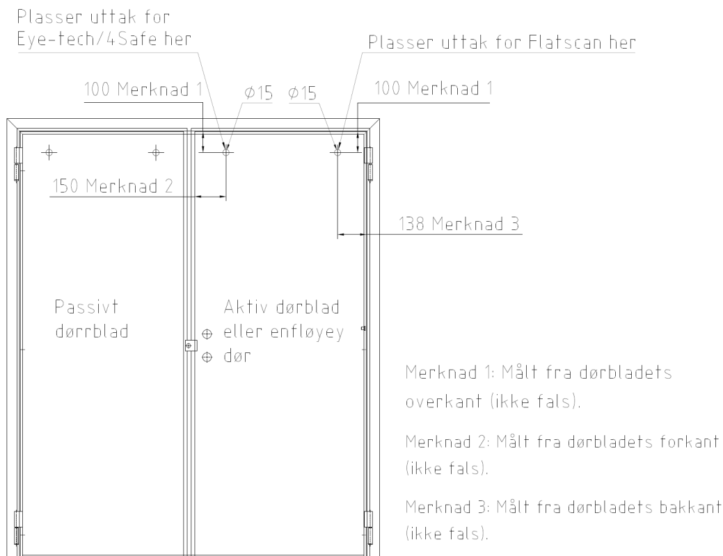
Figur 2. Uttak i dørblad.
